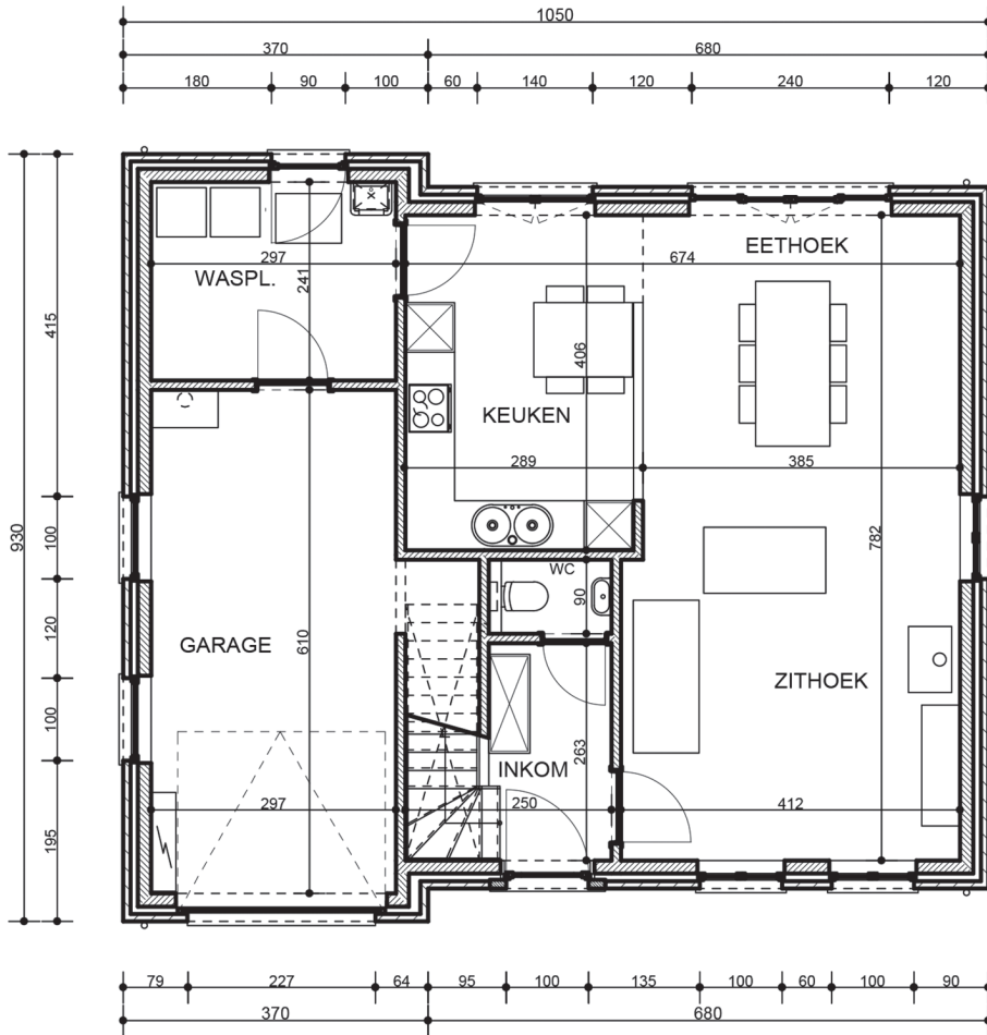
GELIJKVLOERS
