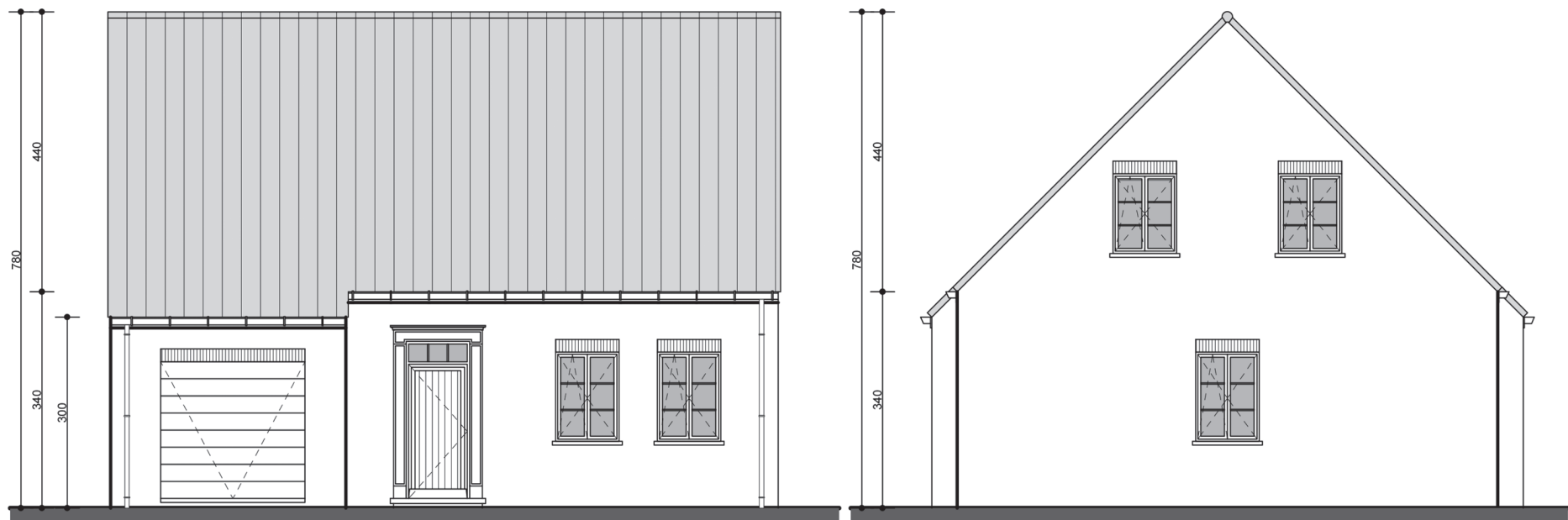
VOORGEVEL
