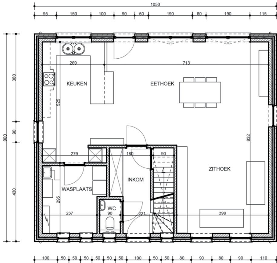
GELIJKVLOERS
