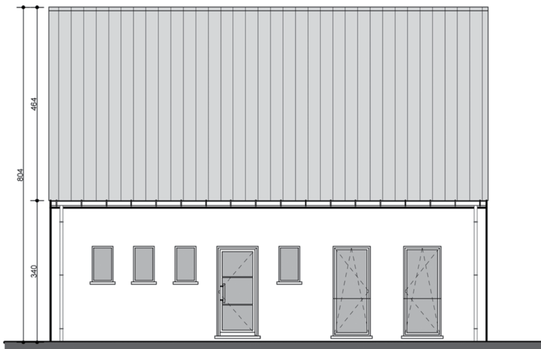
VOORGEVEL
