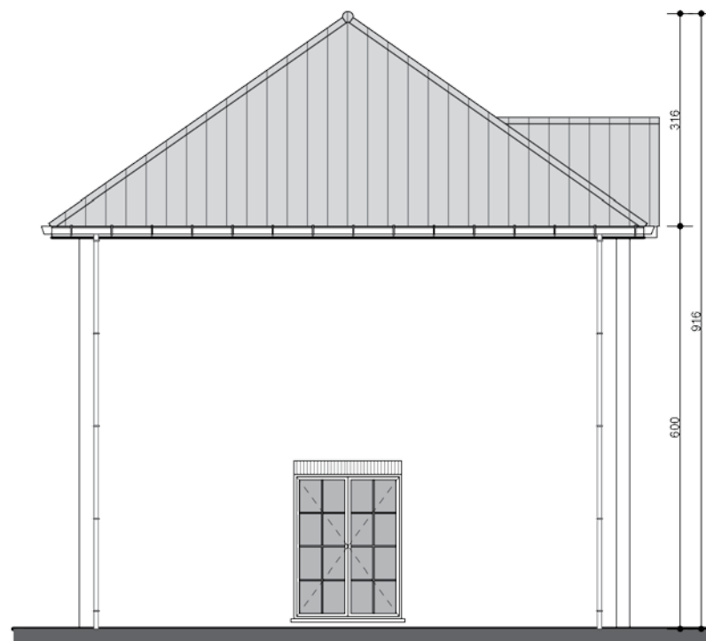
ZIJGEVEL LINKS
