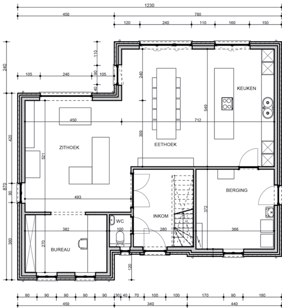
GELIJKVLOERS
