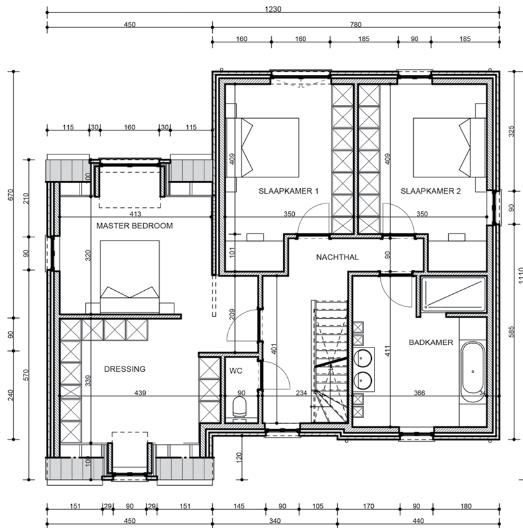
VERDIEPING
