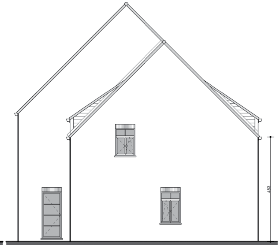
ZIJGEVEL LINKS
