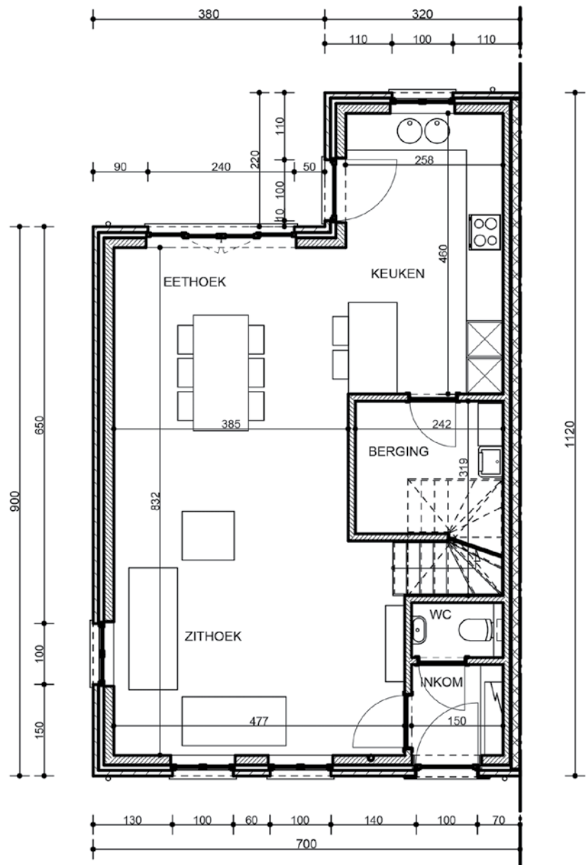
GELIJKVLOERS
