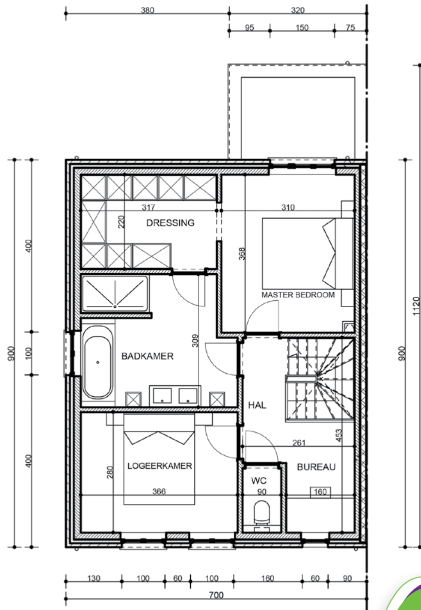
VERDIEPING
