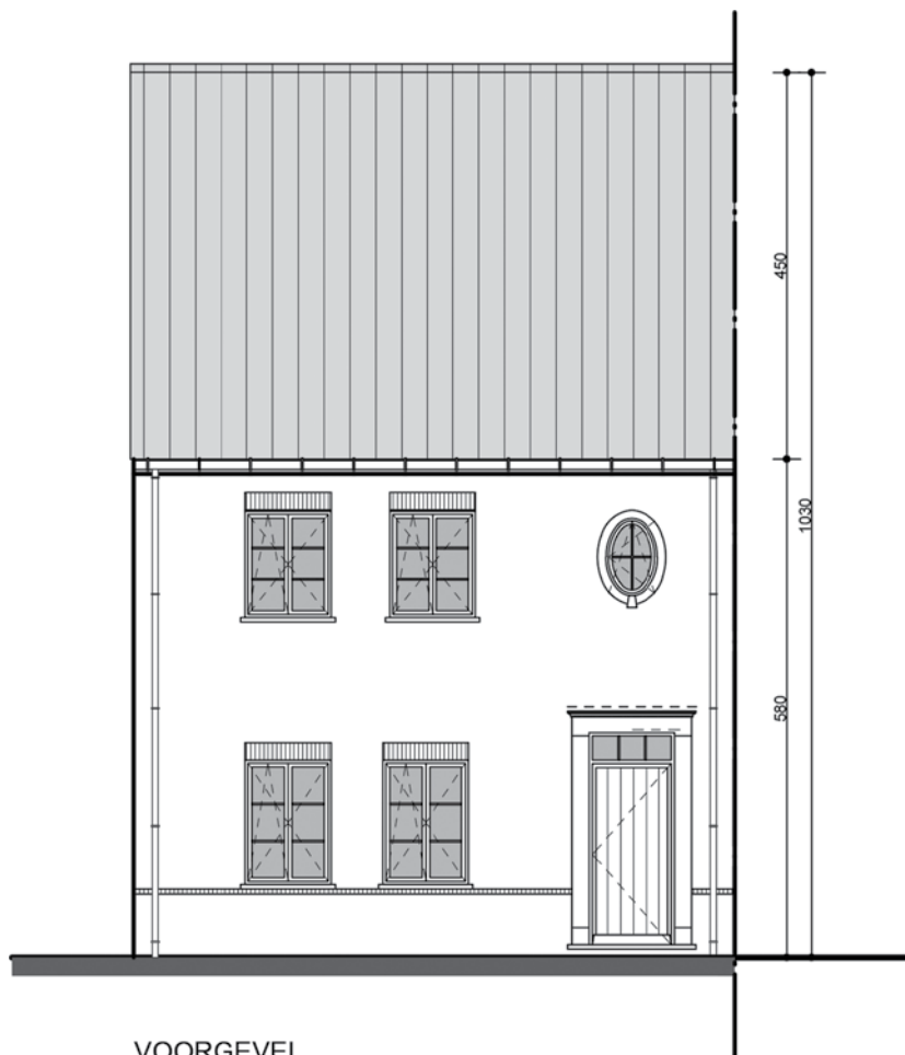
VOORGEVEL
