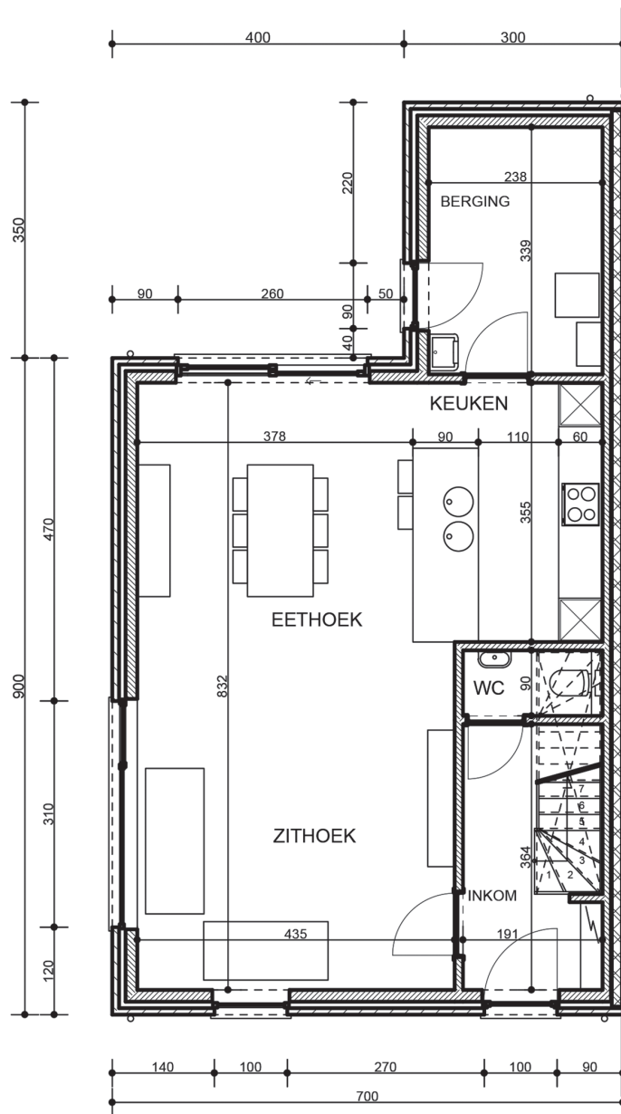
GELIJKVLOERS
