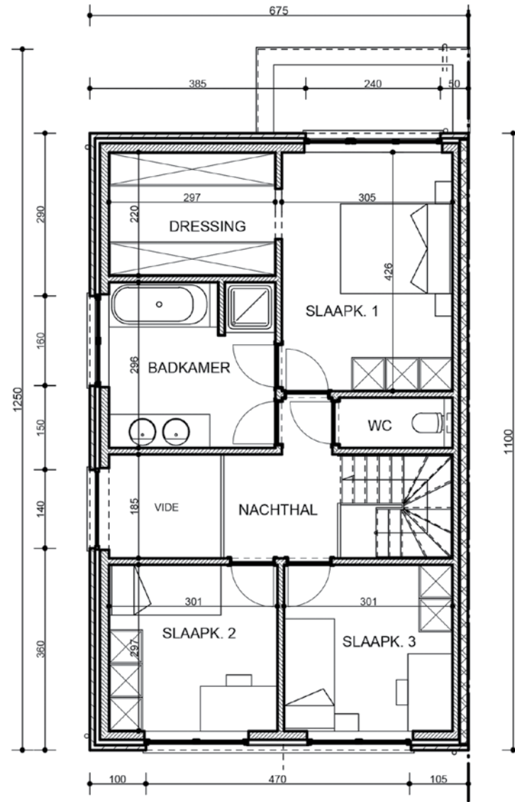
VERDIEPING
