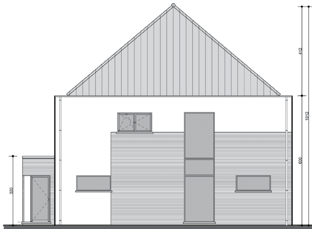
ZIJGEVEL LINKS
