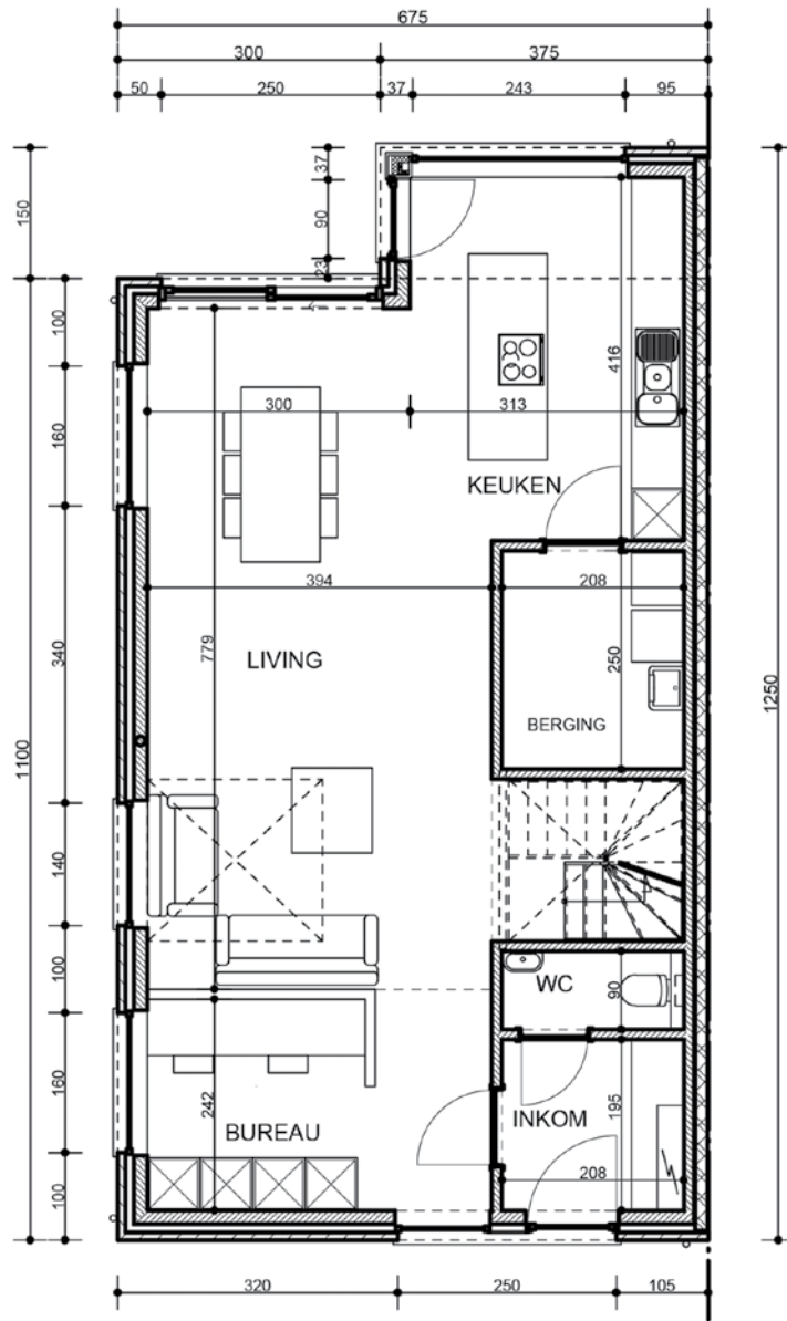
GELIJKVLOERS
